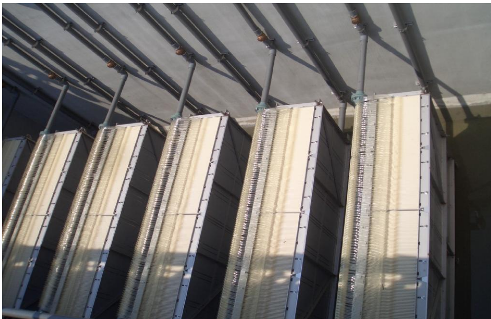
薄膜組在 MBR 槽池中擺設狀況，使用型號為 ES200 R2 總共六組。
